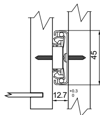
Монтажни размери
